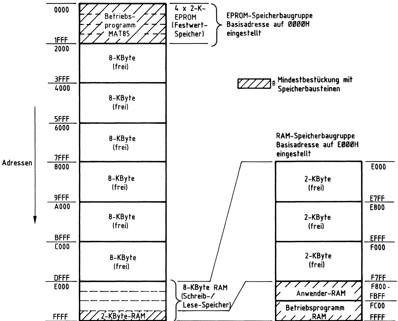
Bild 1: Speicher-Belegung
