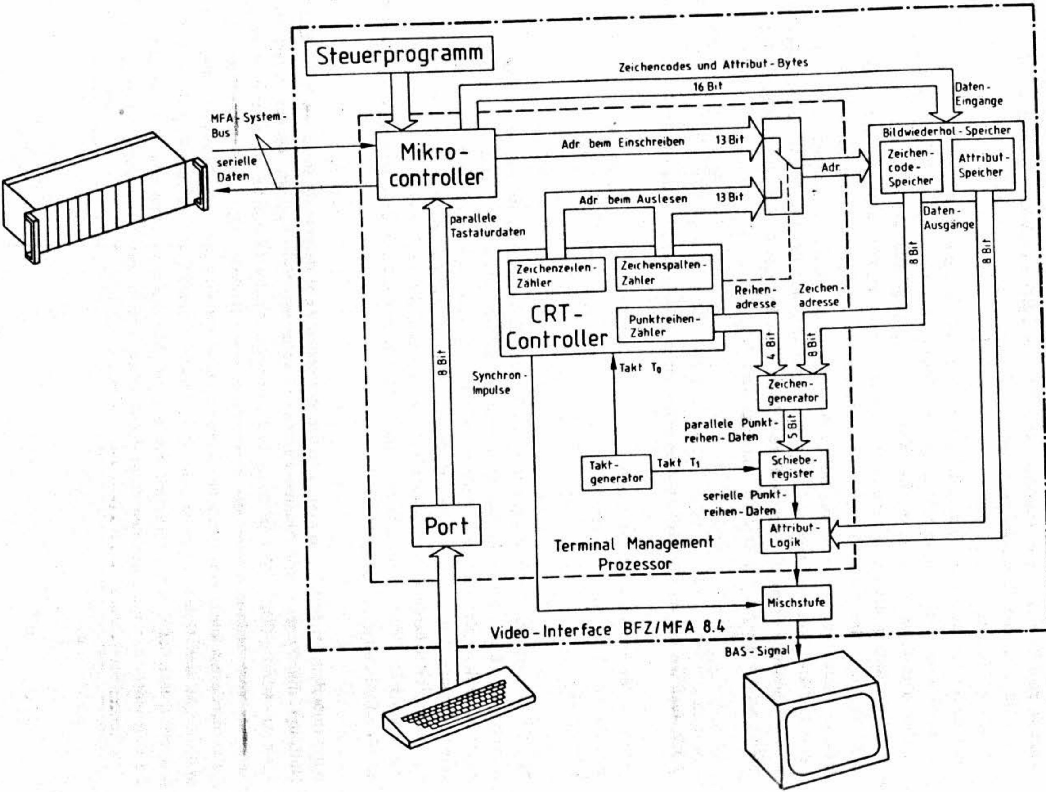
Bild 5: Blockschaltbild des Video-Interfaces
