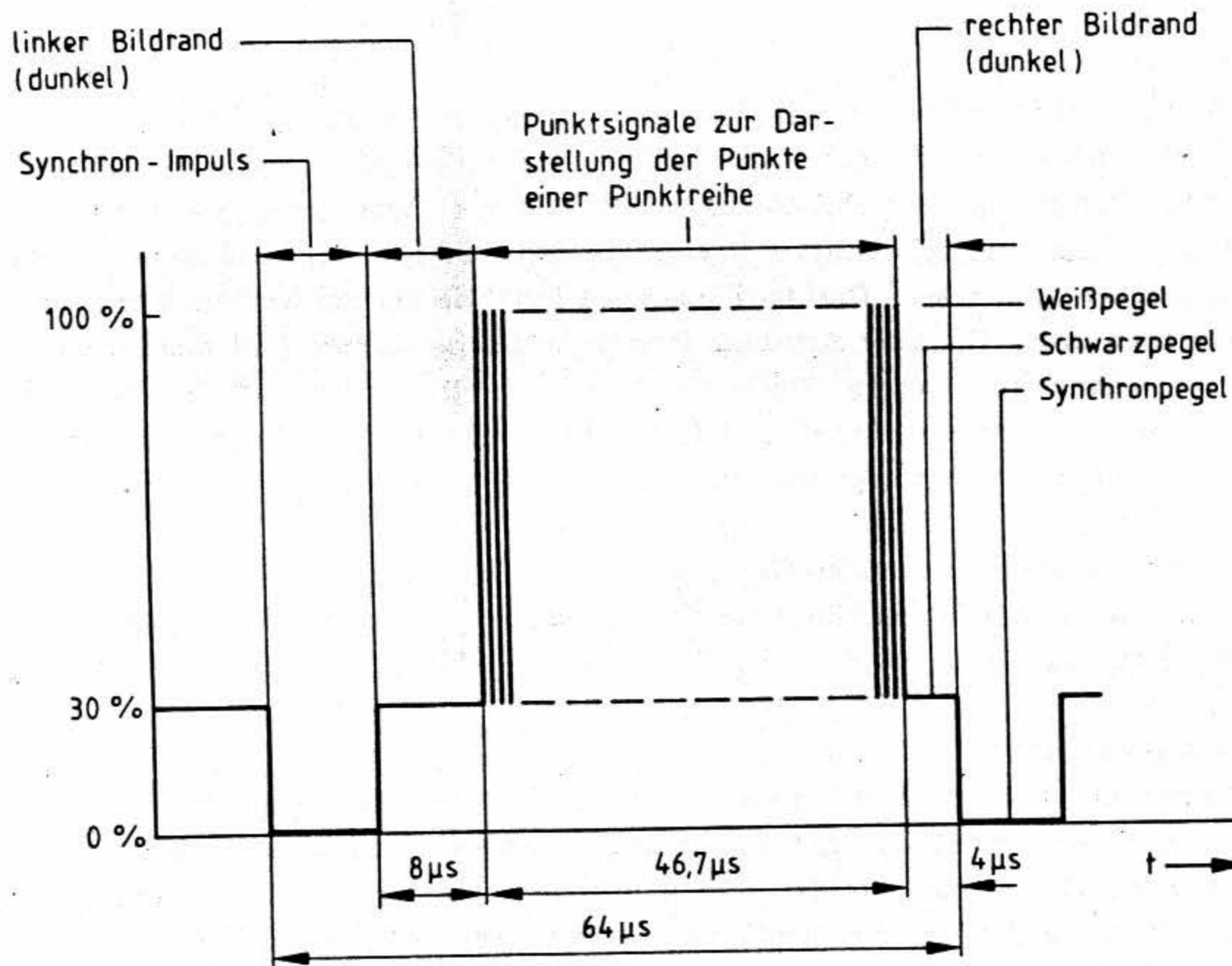
Bild 4: Das BAS-Signal
