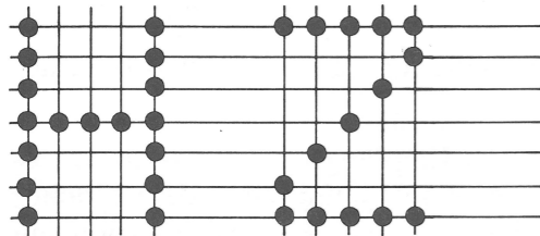
Bild 71: Die Zeichendarstellung im 5 \times 7 -Raster, hier für die Buchstaben H und Z.
